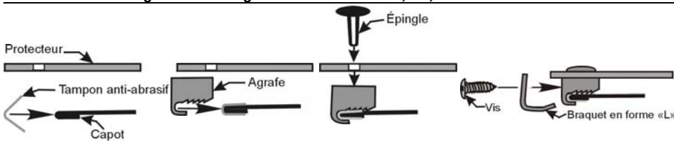
Illustration # 2: Configuration de l'agrafe – No de brevet : 6,892,427
