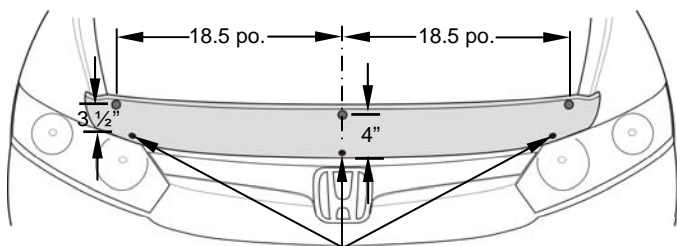
Emplacement des agrafes
